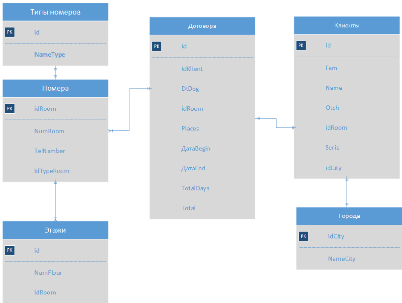
Диаграмма классов – Управление работы с клиентом
