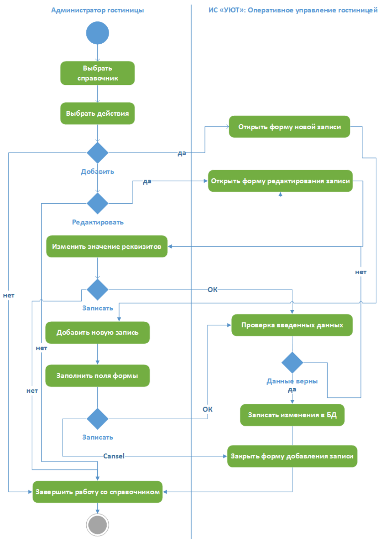
Диаграмма деятельности – Управление справочниками
